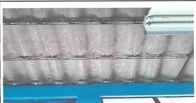
FOTO 6: Techo rajado
